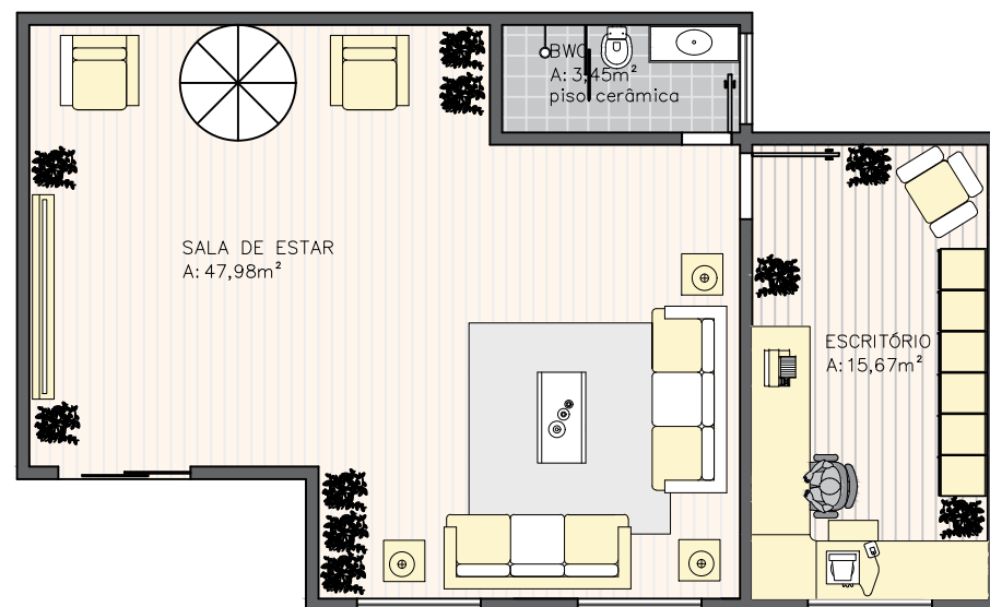
PLANTA LATERAL / DUPLEX TIPO 8, COM 3 QUARTOS 2º PAVIMENTO ÁREA: 73,32m 2
