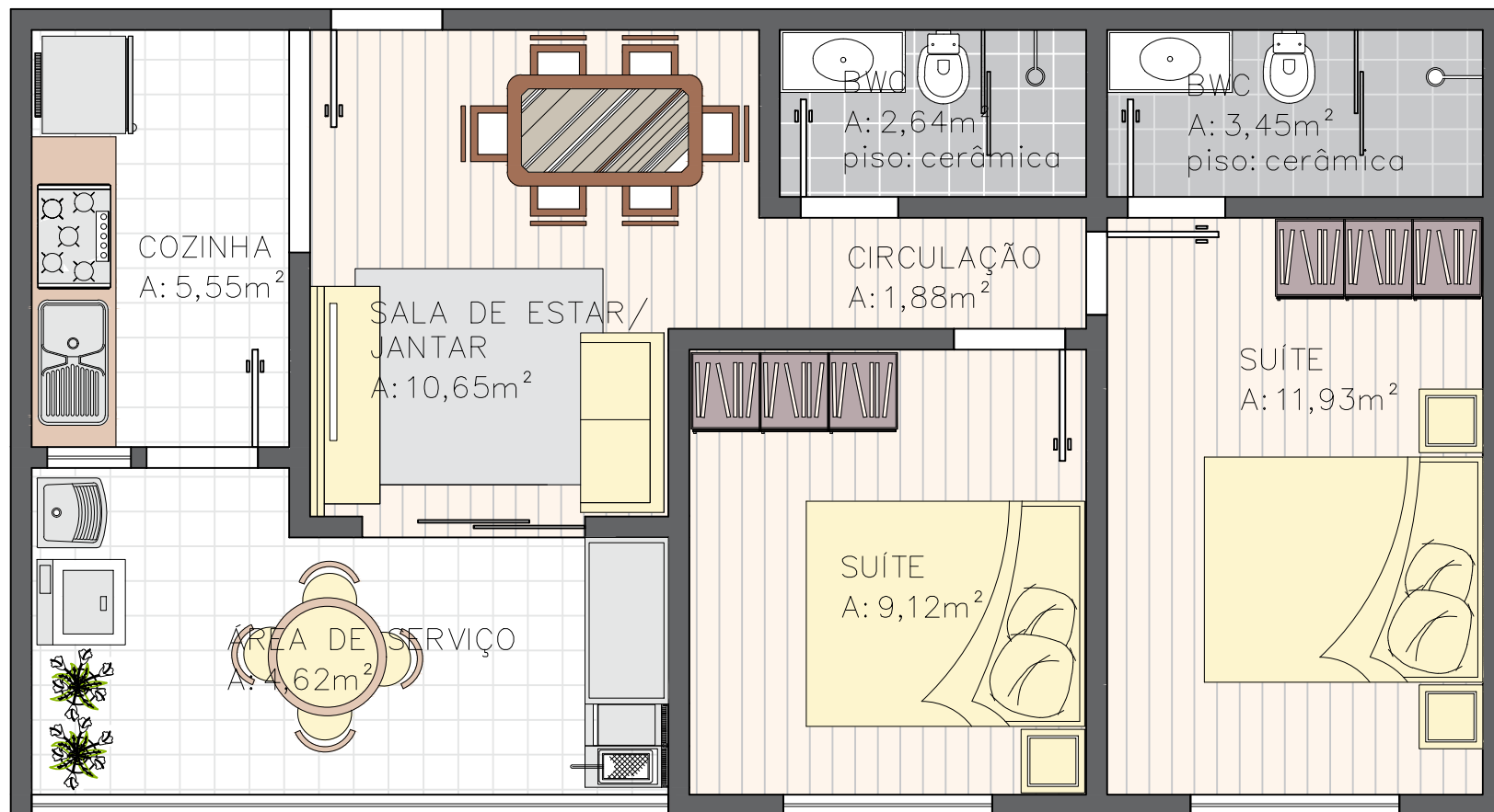
PLANTA MEIO / TIPO 4, COM 2 QUARTOS ÁREA: 62,20m^2
